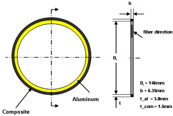
Fig. 6 복합재/알루미늄 링 시편의 형상[13]
