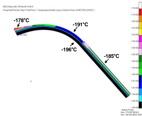
Fig. 2 Type 3 극저온 탱크의 온도 분포
