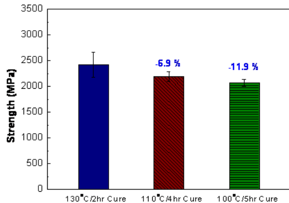
Fig. 9 각 성형온도에서의 복합재/알루미늄 링 시편의 파손 강도
