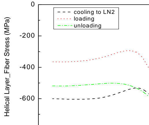
(b) Helical layer 바깥면의 섬유방향응력분포
