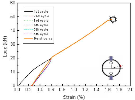
Fig. 8 복합재/알루미늄 링 시편의 하중-변형률 곡선[13]
