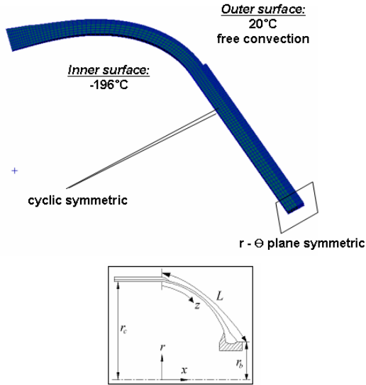
Fig. 1 Type 3 극저온 탱크의 유한요소 모델과 경계조건
